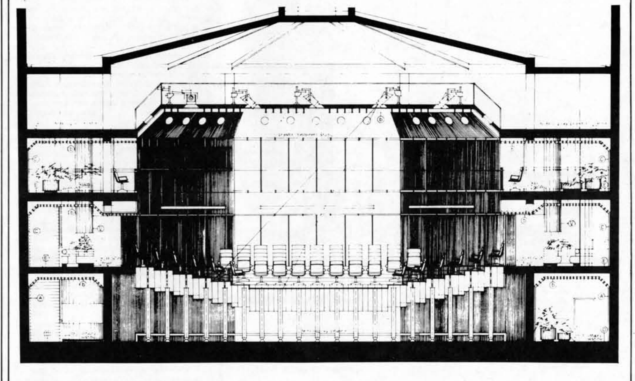
Architektonický návrh Ing. arch. Juraja Hlavicu, Ing. arch. Máriusa Žitňanského, Ing. arch. Štefanie Rosincovej, 1981 – 1983
